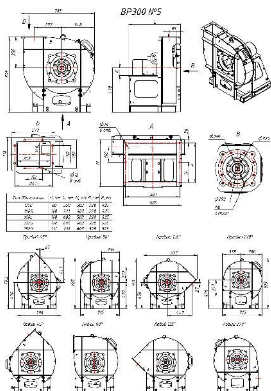
Индустриальный вентилятор BP 300 №5
