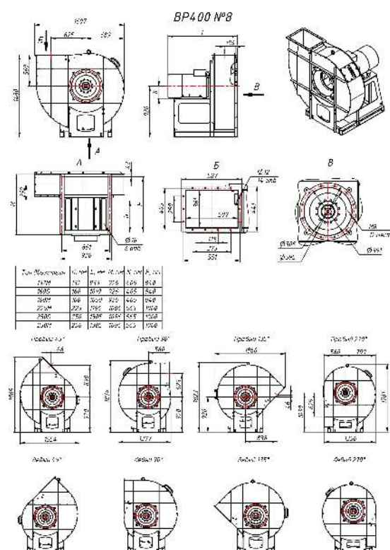
Индустриальный вентилятор BP 400 №8
