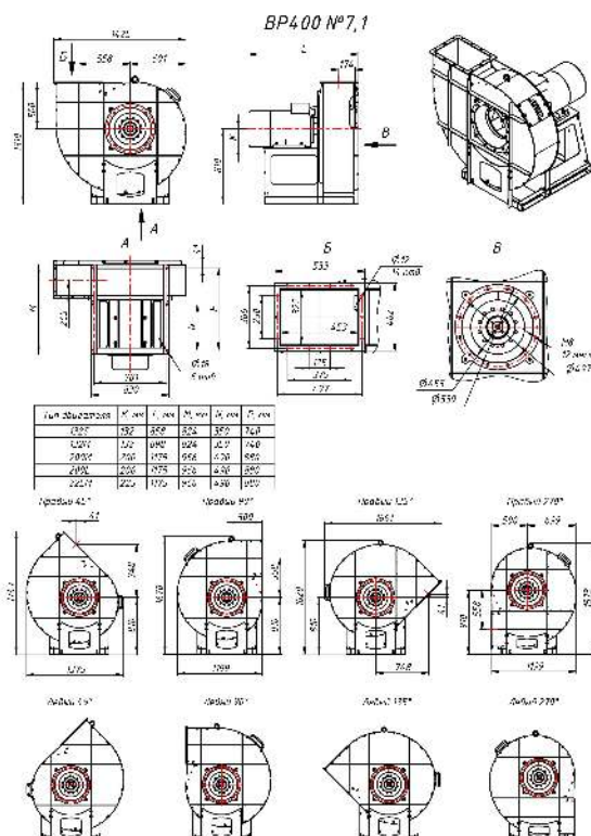
Индустриальный вентилятор BP 400 №7,1
