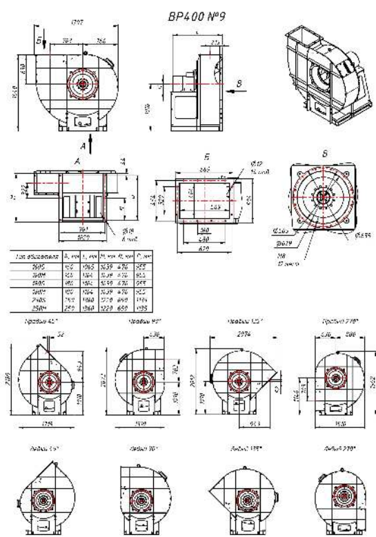
Индустриальный вентилятор BP 400 №9
