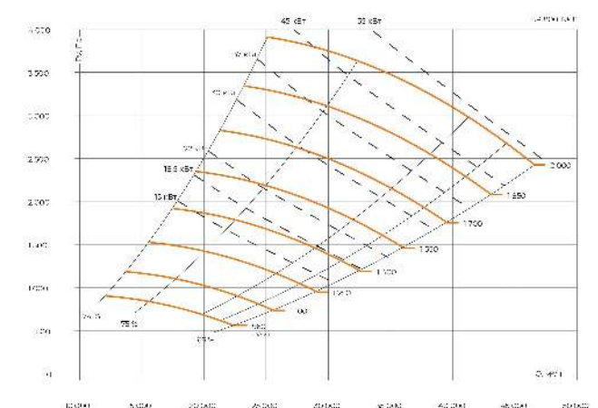
Индустриальный вентилятор BP 800 №8
